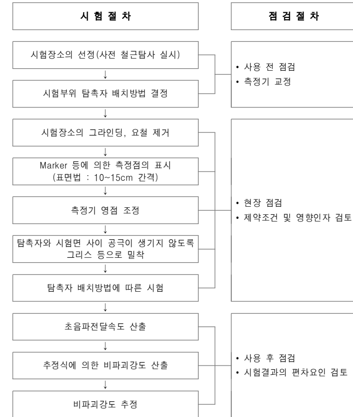
〈그림 3.24〉 초음파전달속도시험 및 측정기 점검 등의 절차
