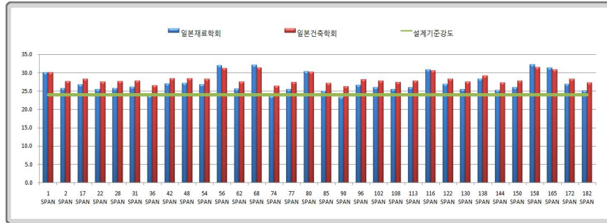
〈그림 3.33〉 터널 라이닝(포항) 평균압축강도 추정결과
