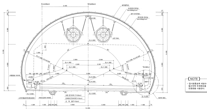
〈표 3.83〉 단면측량(포항) 표준단면도
