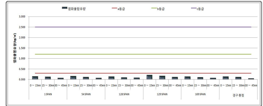
〈그림 3.35〉 염화물함유량 시험결과
