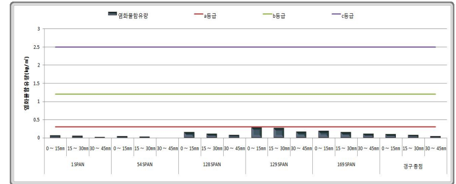
〈그림 3.32〉 염화물함유량 시험결과
