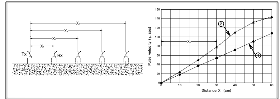
〈그림 3.26〉 표면법에 의한 초음파전달속도의 측정
