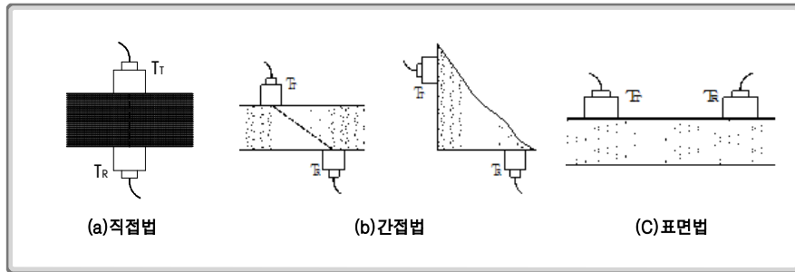
〈그림 3.25〉 초음파전달속도시험을 위한 탐촉자 배치방법
