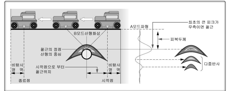
〈그림 3.27〉 철근탐사 측정원리
