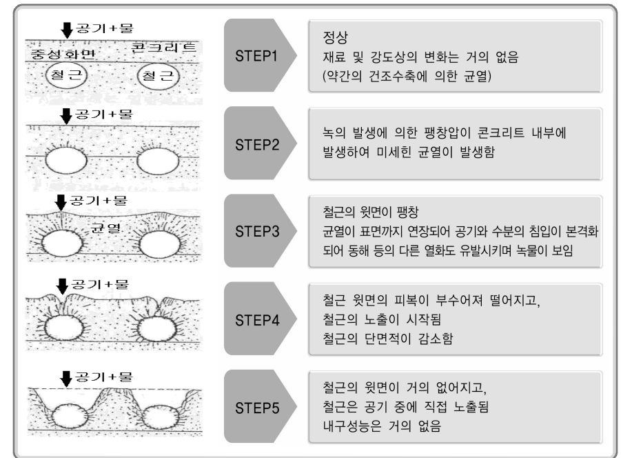
〈그림 3.29〉 탄산화에 의한 철근부식 메카니즘
