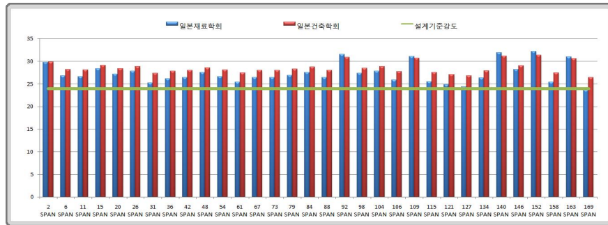
〈그림 3.30〉 터널 라이닝(부산) 평균압축강도 추정결과
