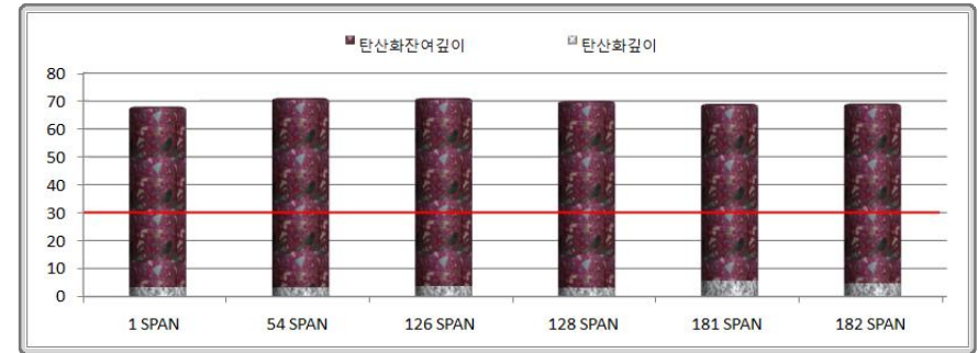
〈그림 3.34〉 탄산화 깊이 측정결과
