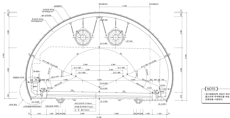
〈표 3.66〉 단면측량(부산) 표준단면도
