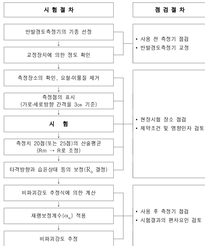
〈그림 3.23〉 반발경도시험 및 측정기 점검 등의 절차
