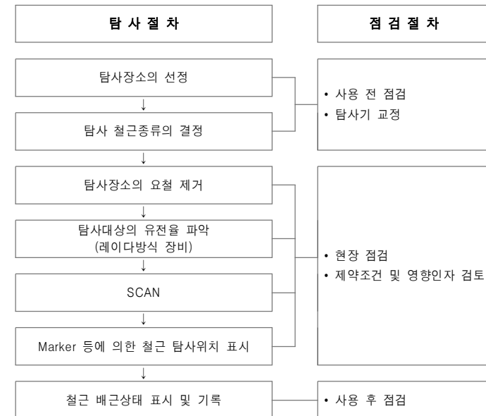
〈그림 3.28〉 철근탐사시험 및 장비 점검 등의 절차
