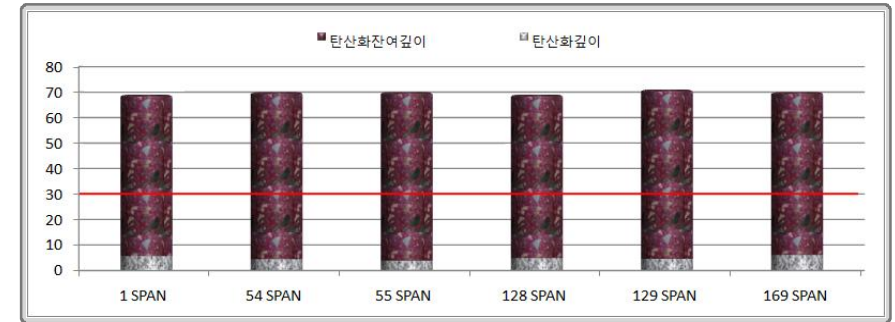
〈그림 3.31〉 탄산화 깊이(부산) 측정결과
